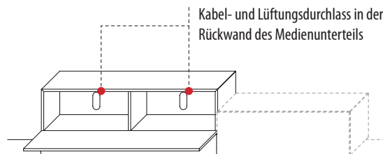
TYPE 1462: Ansicht mit Klappe offen TYPE 1060
