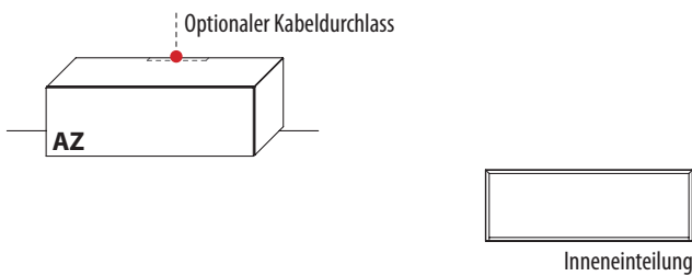
B 105,6 cm x H 37,2 cm x T 44,2 cm
